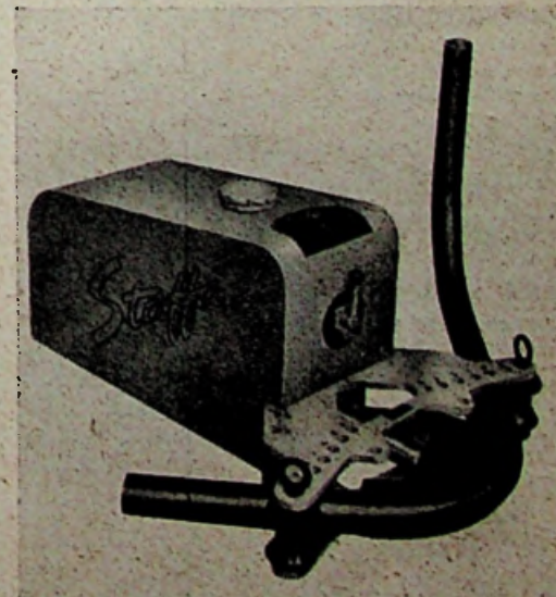
De nieuwe Staffa hydraulische pijp-buigmachine.
